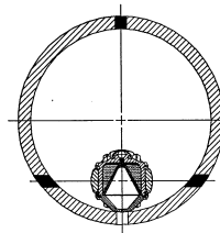
Фазировка 90°
