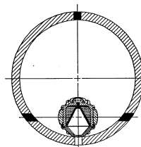
Фазировка 90°
