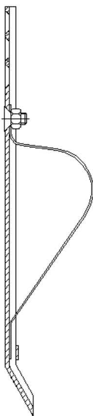
Наконечник STRIP
